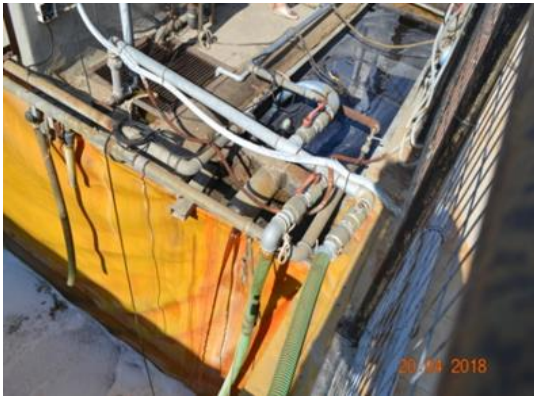
Εικόνα 5: Άποψη της μονάδας επεξεργασίας υγρών αποβλήτων.
