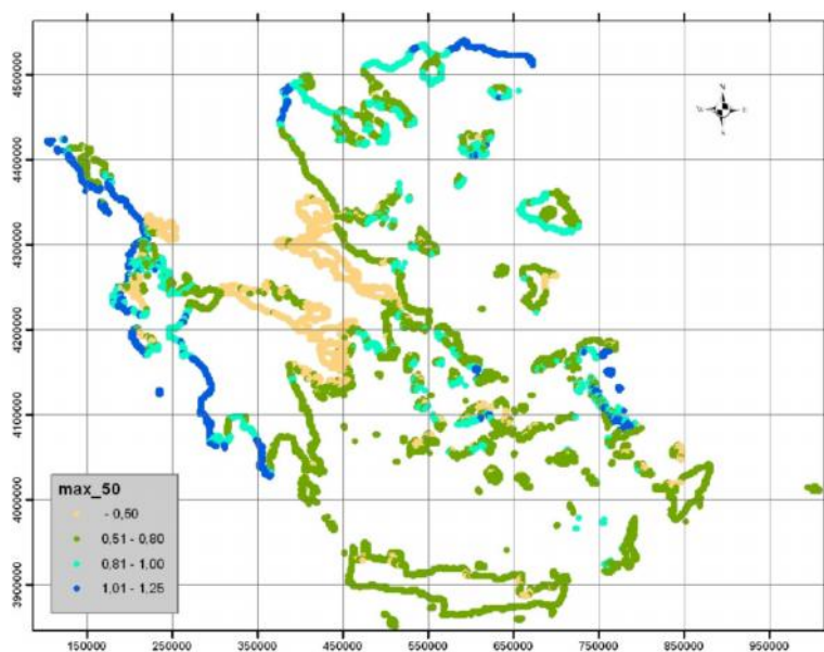
Εικόνα 4-15: Συνολική μέγιστη ανύψωση ΜΣΘ στην ακτογραμμή, από όλες τις διευθύνσεις, για T=50 έτη
