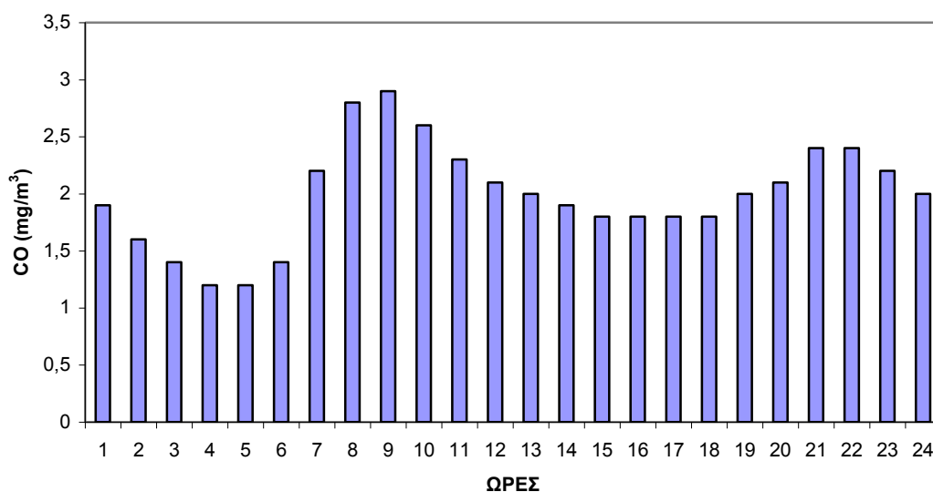
Σχήμα 2.17 Ωριαία μεταβολή CO στο σταθμό Πατησίων για το έτος 2008.
