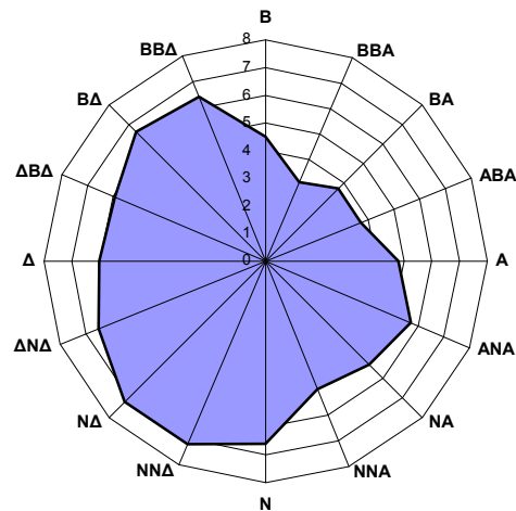
Σχήμα 3.10 Μέσες τιμές βενζολίου (σε \mu\text{g}/\text{m}^3 ) για το έτος 2008 στο σταθμό Πατησίων για κάθε διεύθυνση του ανέμου.
