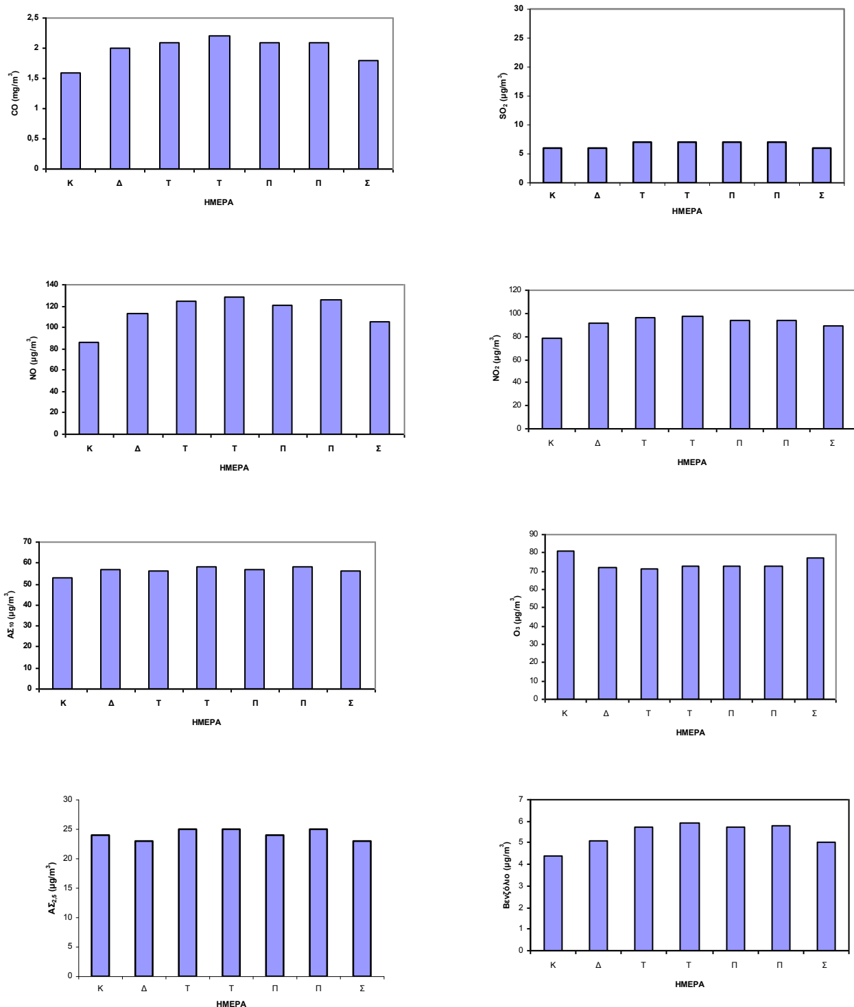
Σχήμα 2.16 Ημερήσια μεταβολή συγκεντρώσεων CO, NO, NO 2 και βενζολίου στο σταθμό Πατησίων, SO 2 στο σταθμό Γεωπονική, ΔΣ 10 στο σταθμό Αριστοτέλους, ΑΣ 2,5 στο σταθμό Γουδή, και O 3 στο σταθμό Λυκόβρυση για το έτος 2008.
