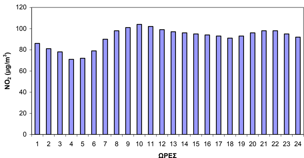
Σχήμα 2.21 Ωραία μεταβολή NO 2 στο σταθμό Πατησίων για το έτος 2008.
