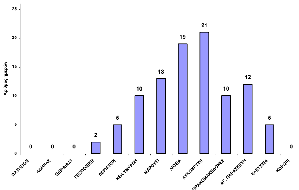
Σχήμα 5.2 Αριθμός ημερών για το 2008 με ωριαία τιμή όζοντος μεγαλύτερη από 180 \mu\text{g}/\text{m}^3
