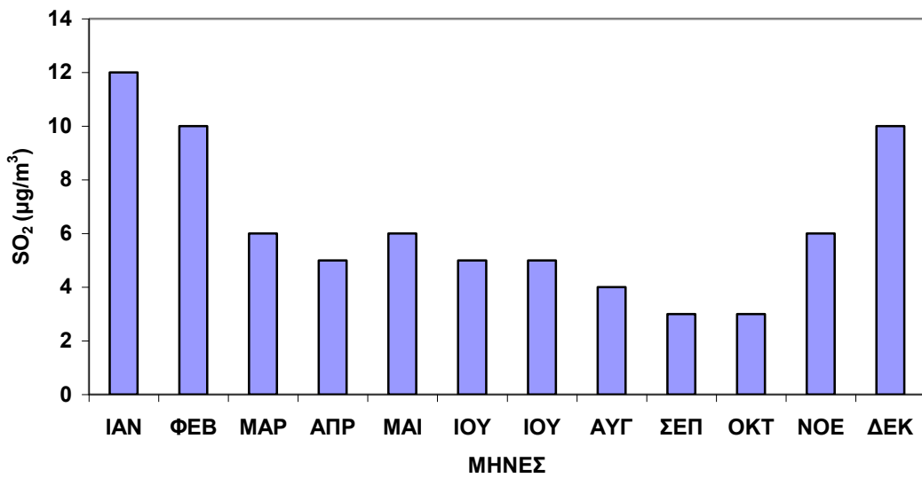
Σχήμα 2.9. Μέσες μηνιαίες τιμές SO 2 στο σταθμό Γεωπονική για το έτος 2008.
