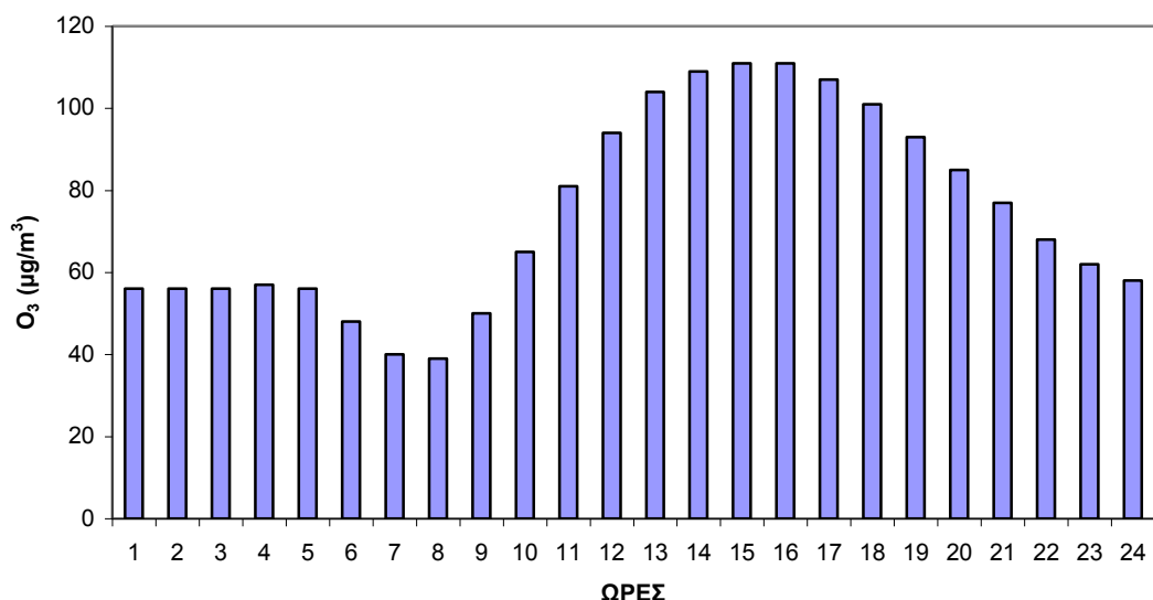
Σχήμα 2.22 Ωραία μεταβολή O 3 στο σταθμό Λυκόβρυση για το έτος 2008.
