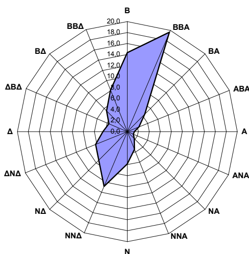
Σχήμα 3.1 Συχνότητες, επί τοις εκατό (%), των διευθύνσεων του ανέμου στο σταθμό Πατησίων για το έτος 2008.
