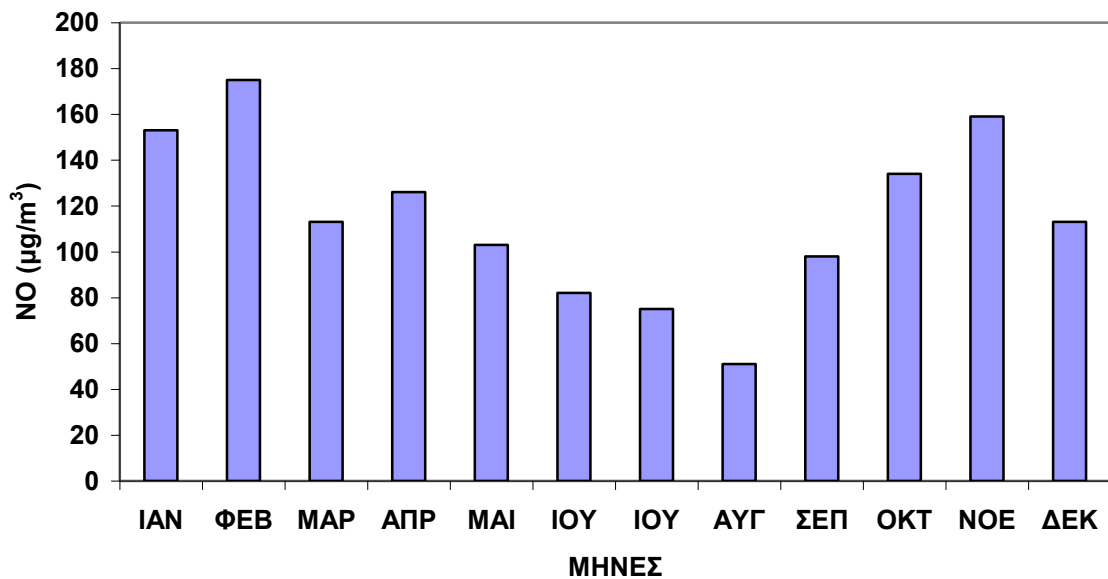
Σχήμα 2.11. Μέσες μηνιαίες τιμές NO 2 στο σταθμό Πατησίων για το έτος 2008.
