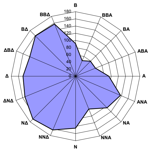
Σχήμα 3.6 Μέσες τιμές NO (σε \mu\text{g}/\text{m}^3 ) για το έτος 2008 στο σταθμό Πατησίων για κάθε διεύθυνση του ανέμου.
