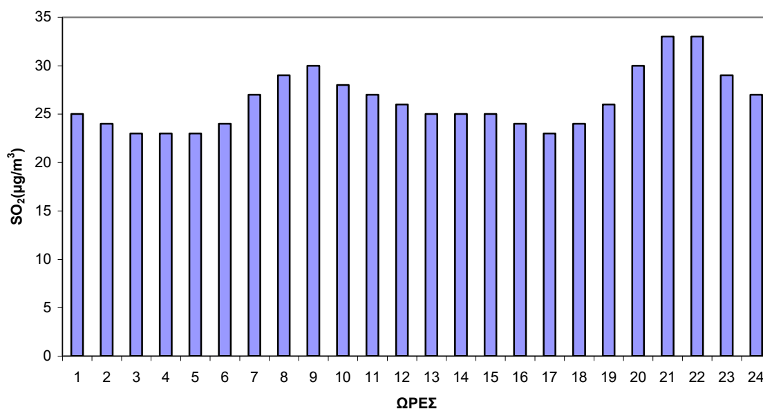
Σχήμα 2.18 Ωριαία μεταβολή SO 2 στο σταθμό Πατησίων για το έτος 2008.
