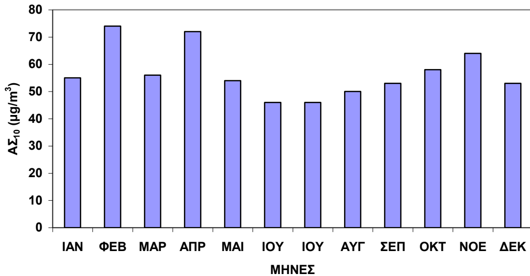
Σχήμα 2.13. Μέσες μηνιαίες τιμές ΑΣ 10 στο σταθμό Αριστοτέλους για το έτος 2008.
