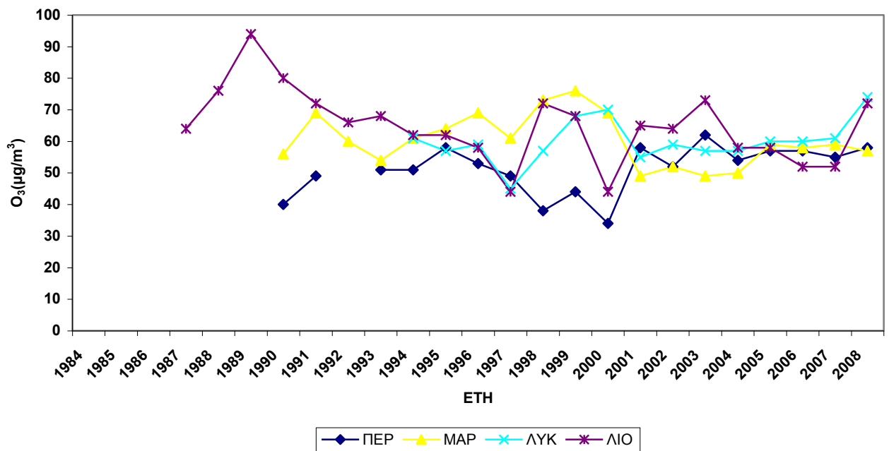
Σχήμα 2.6.β Διαχρονική μεταβολή μέσω των ετήσιων τιμών O 3 , σε µg/m 3 .
