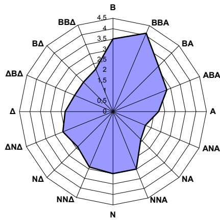
Σχήμα 3.2 Μέση ταχύτητα ανά διεύθυνση ανέμου, στο σταθμό Πατησίων για το έτος 2008
