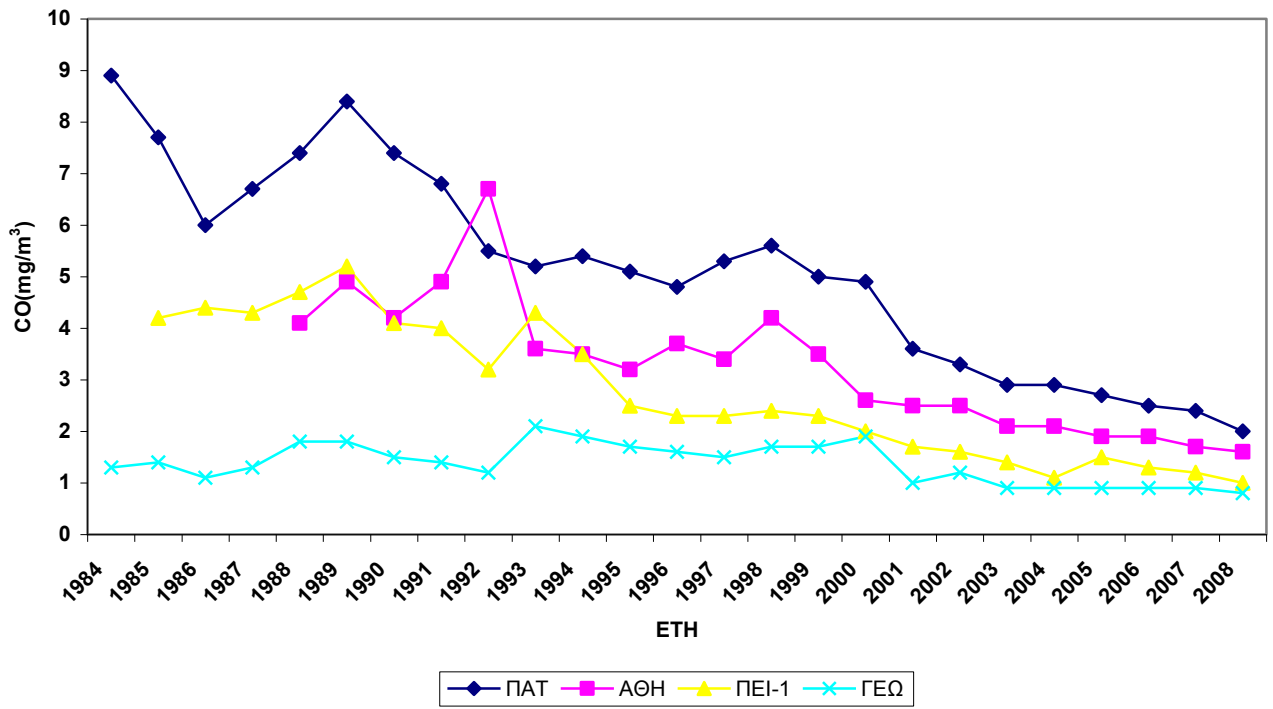
Σχήμα 2.1.α Διαχρονική μεταβολή μέσωσν ετησίωσν τιμών CO, σε mg/m 3 .
