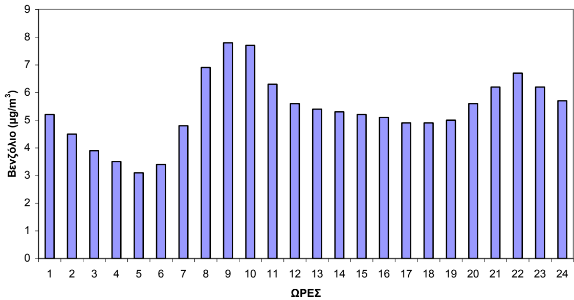
Σχήμα 2.20 Ωριαία μεταβολή βενζολίου στο σταθμό Πατησίων για το έτος 2008.
