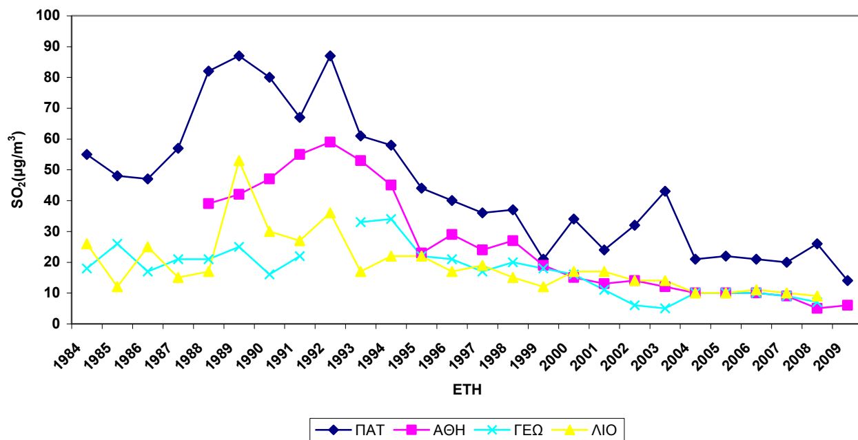
Σχήμα 2.2.α Διαχρονική μεταβολή μέσων ετήσιων τιμών SO_2 σε \mu g/m^3 .
