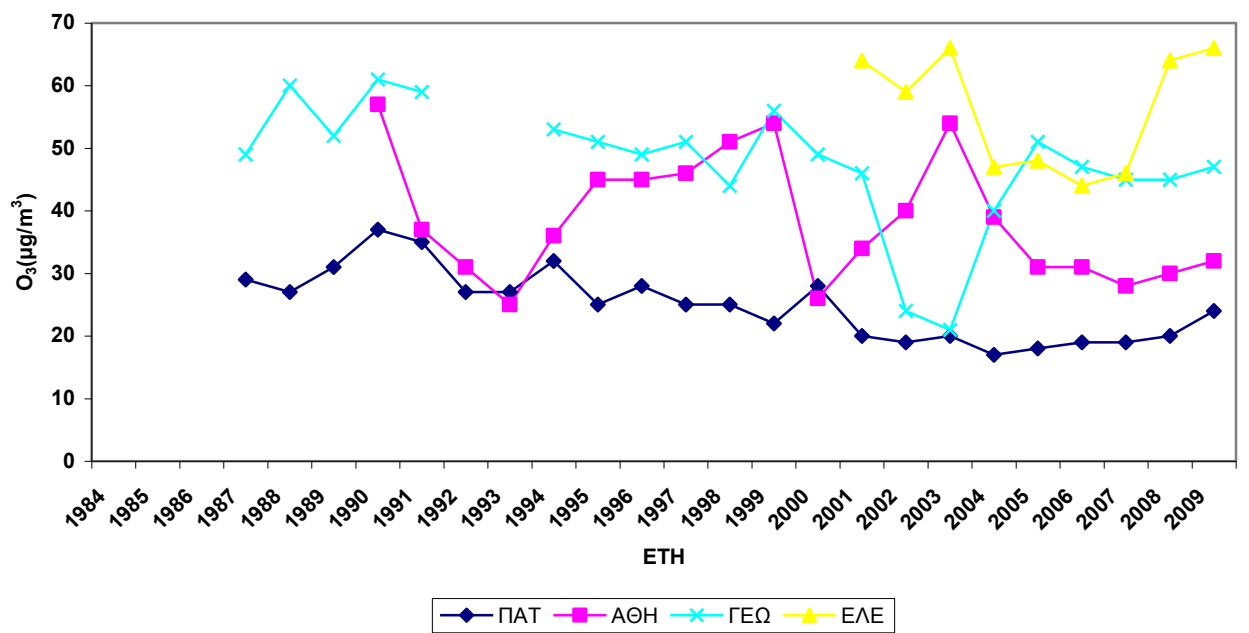
Σχήμα 2.6.α Διαχρονική μεταβολή μέσων ετήσιων τιμών \text{O}_3 , σε \mu\text{g}/\text{m}^3 .
