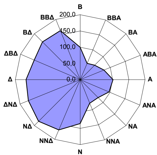
Σχήμα 3.6 Μέσες τιμές NO (σε \mu\text{g}/\text{m}^3 ) για το έτος 2009 στο σταθμό Πατησίων για κάθε διεύθυνση του ανέμου.
