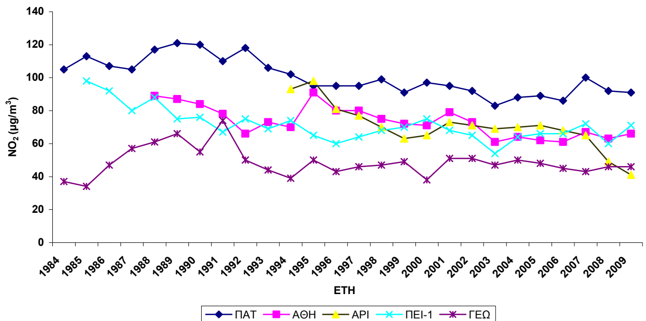
Σχήμα 2.5.α Διαχρονική μεταβολή μέσων ετήσιων τιμών NO 2 , σε \mu\text{g}/\text{m}^3 .
