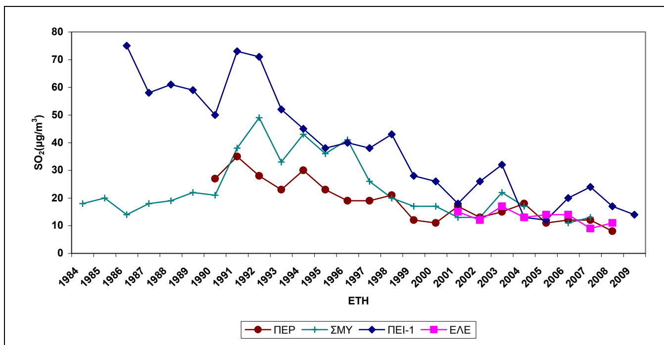
Σχήμα 2.2.β Διαχρονική μεταβολή μέσων ετήσιων τιμών SO_2 σε \mu g/m^3 .
