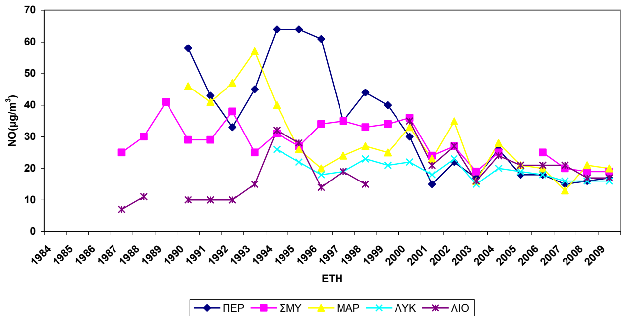
Σχήμα 2.4.β Διαχρονική μεταβολή μέσων ετήσιων τιμών NO σε \mu\text{g}/\text{m}^3 .
