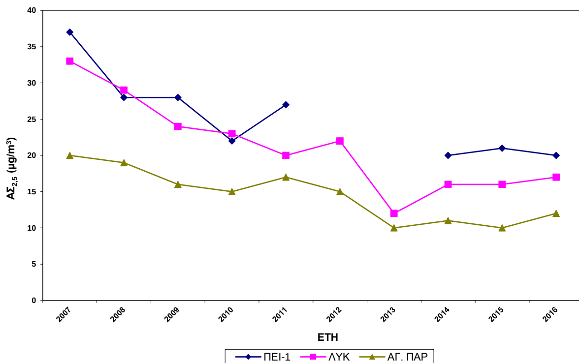
Σχήμα 2.8. Διαχρονική μεταβολή μέσων ετήσιων τιμών AS_{2.5} , σε \mu g/m^3 .
