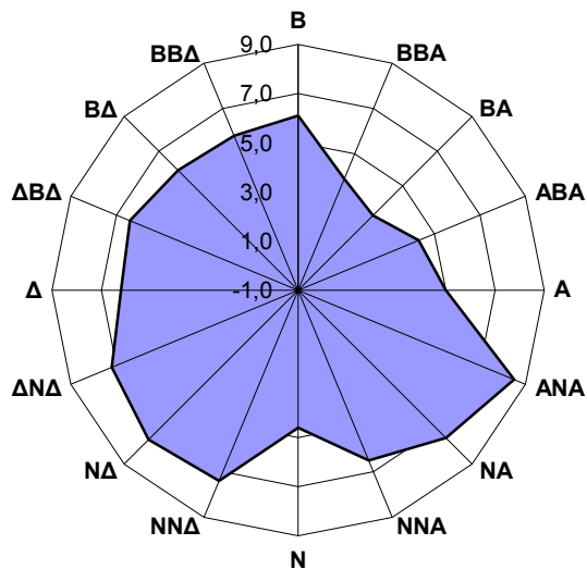
Σχήμα 3.10 Μέσες τιμές βενζολίου (σε \mu\text{g}/\text{m}^3 ) για το έτος 2016 στο σταθμό Πατησίων για κάθε διεύθυνση του ανέμου.
