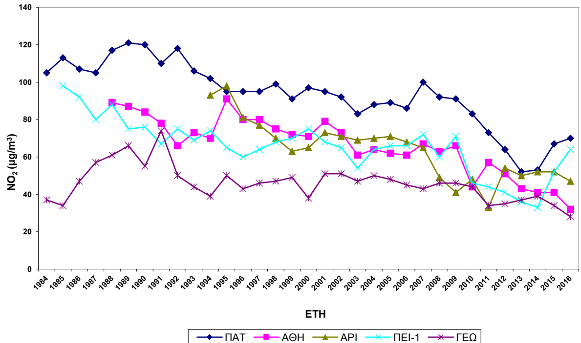
Σχήμα 2.5.α Διαχρονική μεταβολή μέσων ετήσιων τιμών \text{NO}_2 , σε \mu\text{g}/\text{m}^3 .
