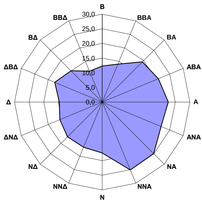
Σχήμα 3.9 Μέσες τιμές AS_{2.5} (σε \mu g/m^3 ) για το έτος 2016 στο σταθμό Λυκόβρυση για κάθε διεύθυνση του ανέμου.
