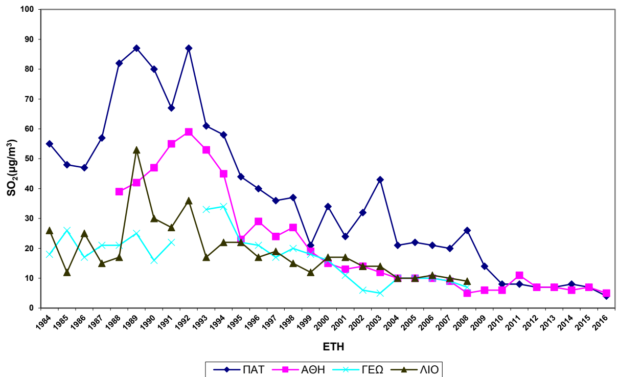
Σχήμα 2.2.α Διαχρονική μεταβολή μέσων ετήσιων τιμών SO_2 , σε \mu g/m^3 .
