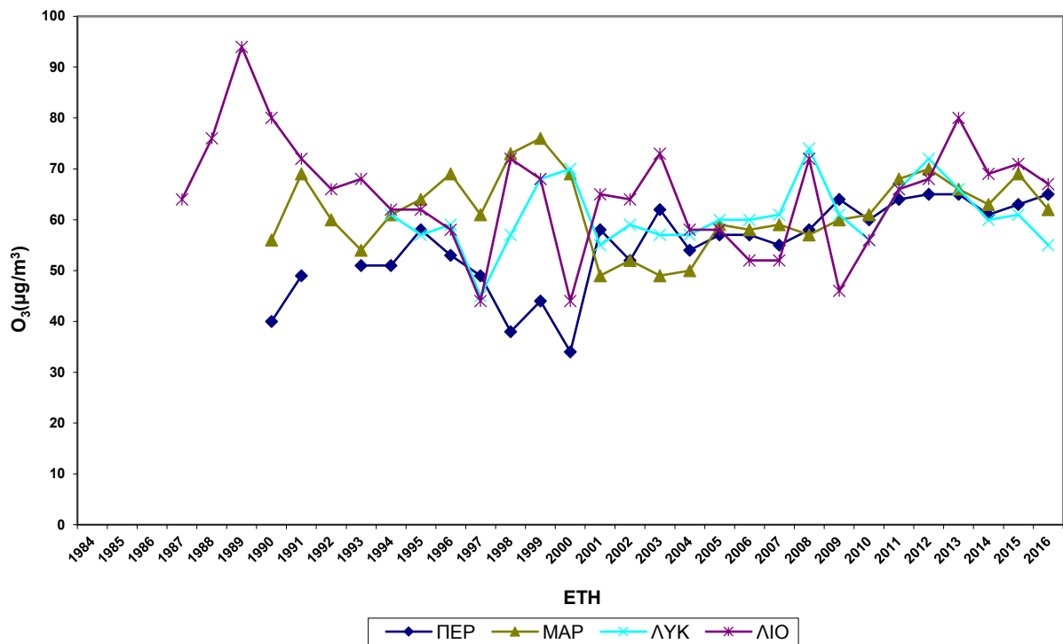
Σχήμα 2.6.β Διαχρονική μεταβολή μέσω των ετήσιων τιμών O_3 , σε \mu g/m^3 .
