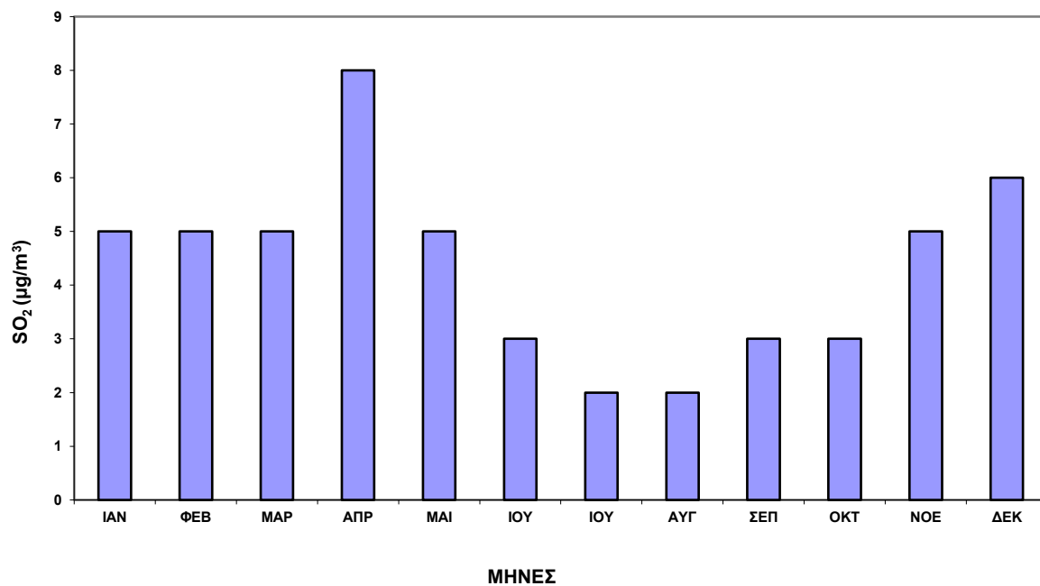
Σχήμα 2.10. Μέσες μηνιαίες τιμές SO 2 στο σταθμό Πατησίων για το έτος 2016.
