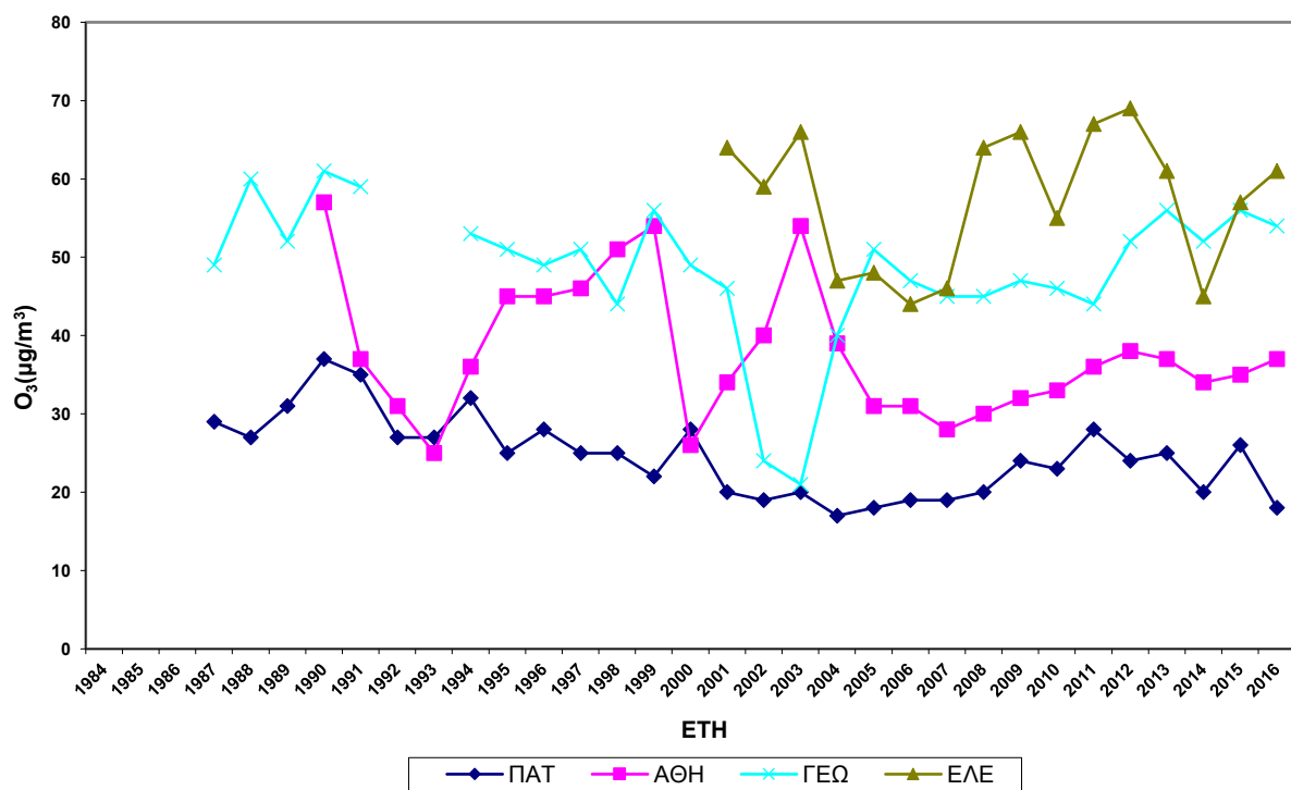
Σχήμα 2.6.α Διαχρονική μεταβολή μέσων ετήσιων τιμών \text{O}_3 , σε \mu\text{g}/\text{m}^3 .
