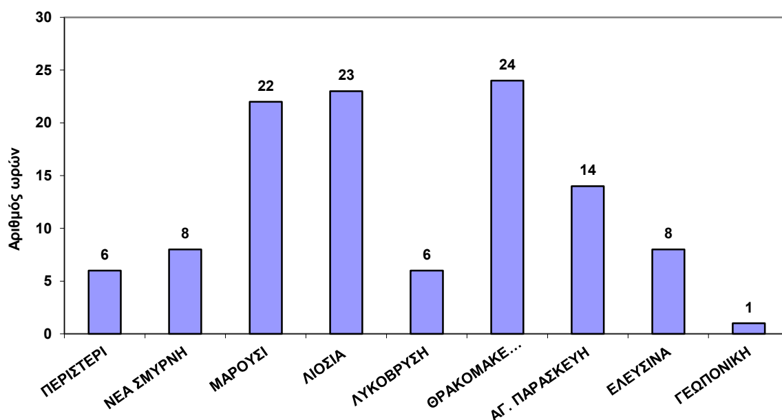
Σχήμα 5.2 Αριθμός ωρών για το 2016 με ωριαία τιμή όζοντος μεγαλύτερη από 180 µg/m 3
