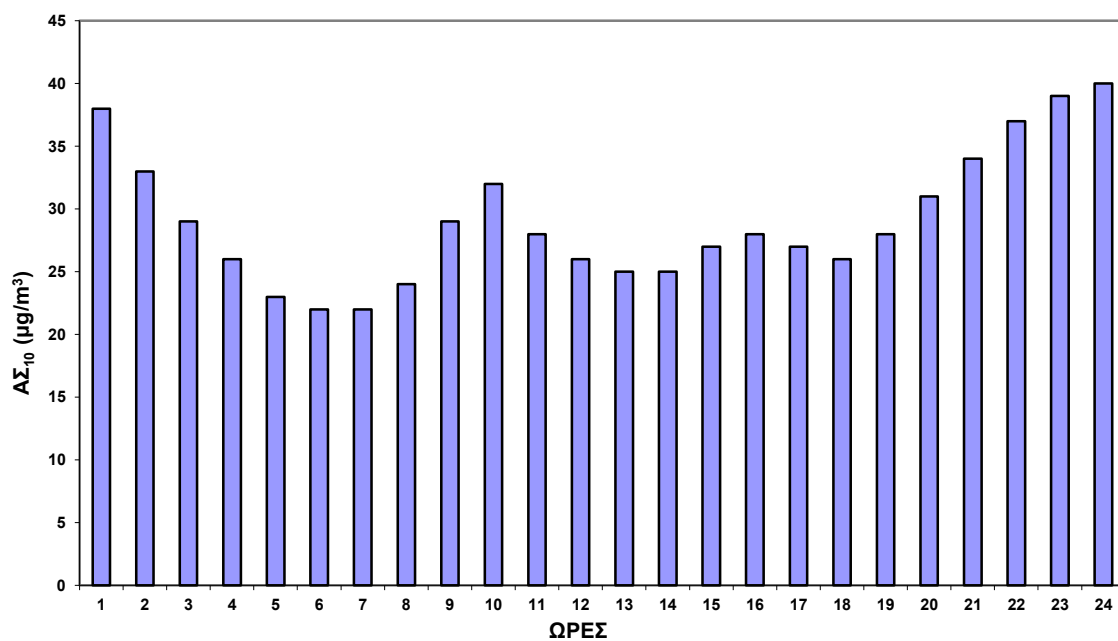
Σχήμα 2.24 Ωριαία μεταβολή AΣ 10 στο σταθμό Λυκόβρυση για το έτος 2016.
