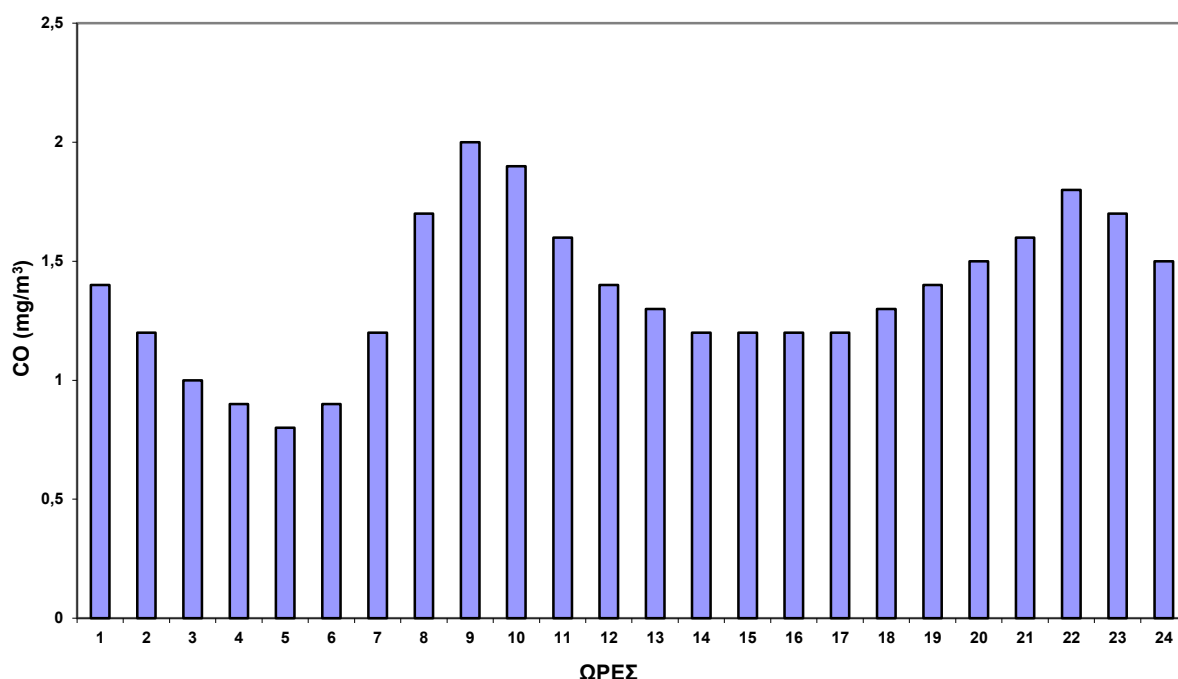
Σχήμα 2.18 Ωριαία μεταβολή CO στο σταθμό Πατησίων για το έτος 2016.
