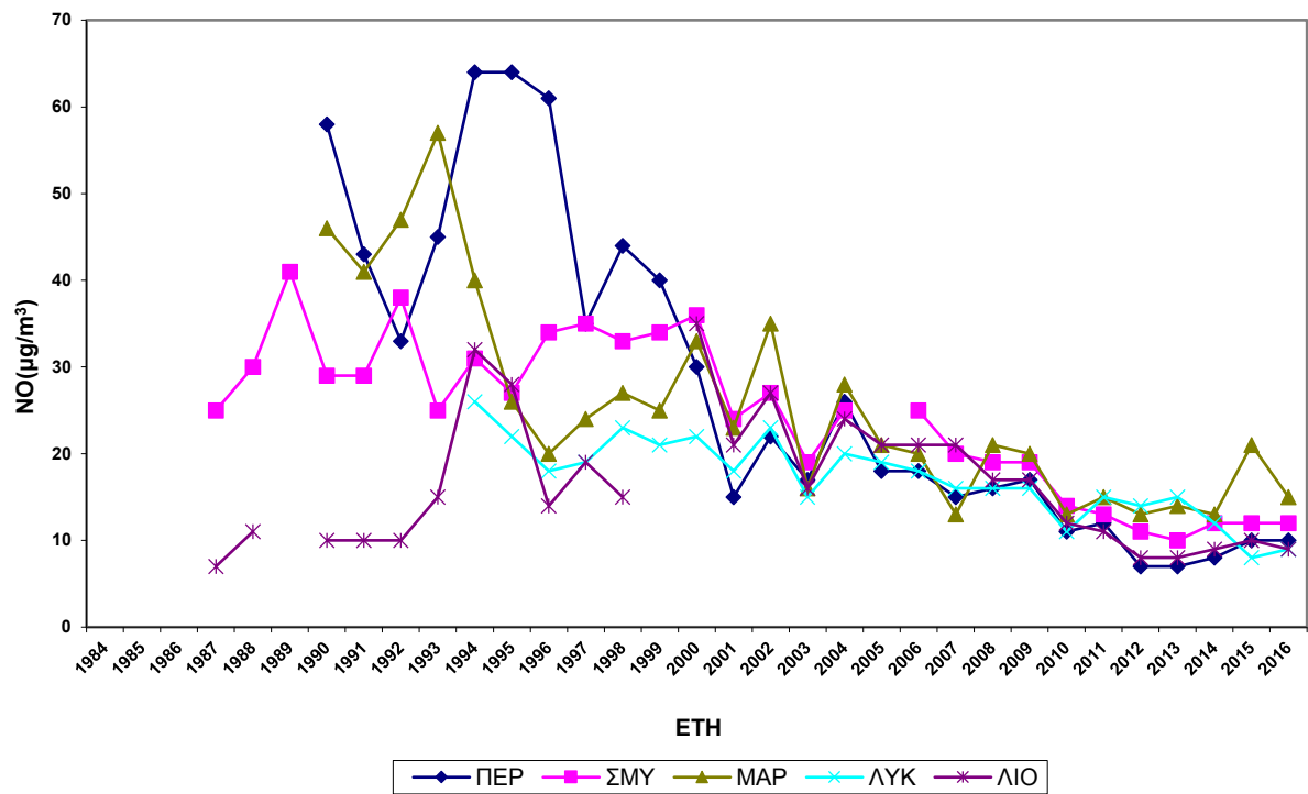
Σχήμα 2.4.β Διαχρονική μεταβολή μέσων ετήσιων τιμών \text{NO} , σε \mu\text{g}/\text{m}^3 .
