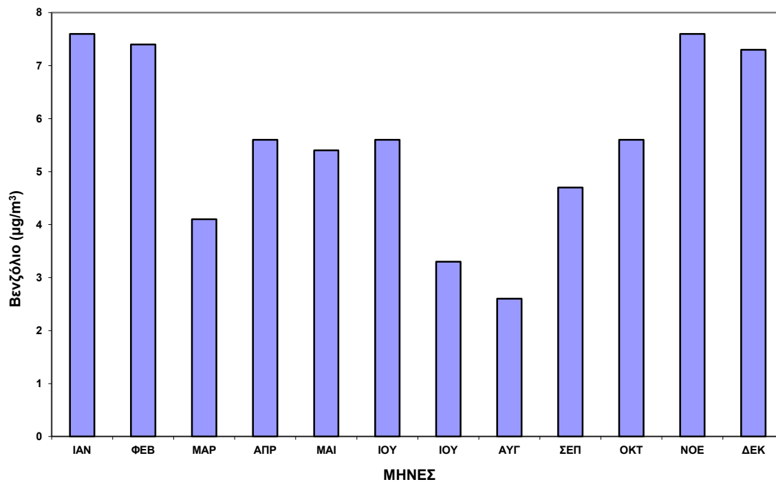
Σχήμα 2.16. Μέσες μηνιαίες τιμές βενζολίου στο σταθμό Πατησίων για το έτος 2016.
