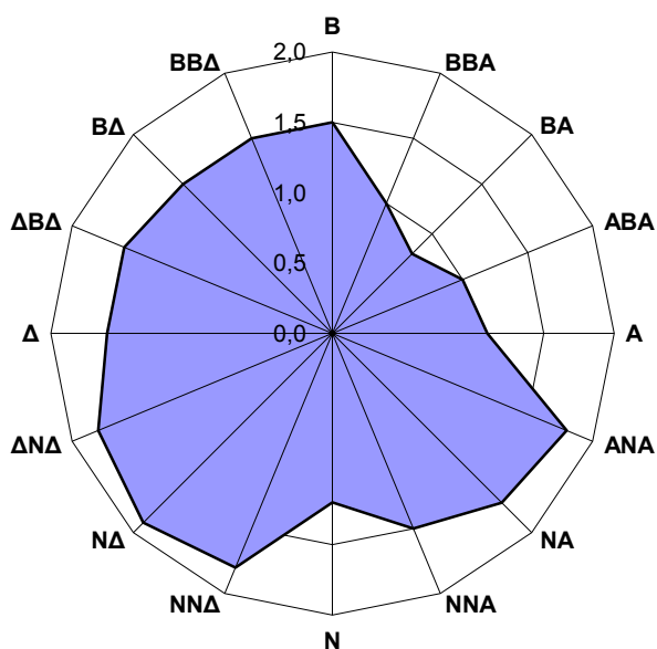
Σχήμα 3.5 Μέσες τιμές CO (σε mg/m 3 ) για το έτος 2016 στο σταθμό Πατησίων για κάθε διεύθυνση του ανέμου.
