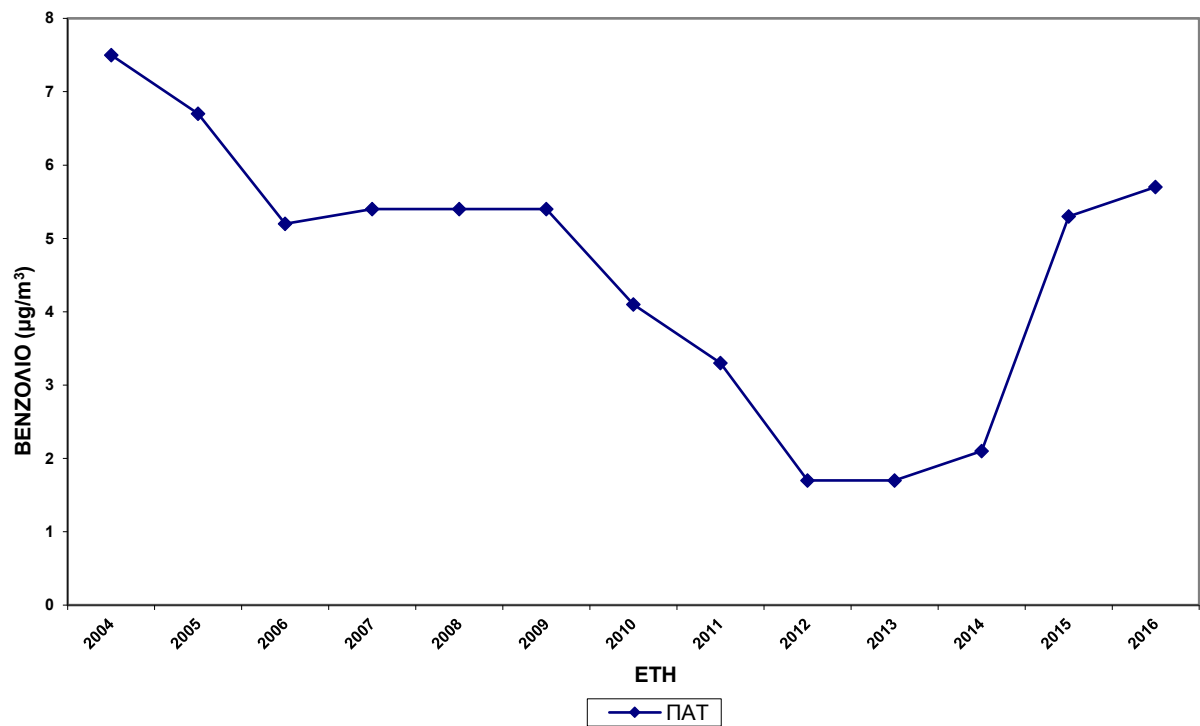
Σχήμα 2.3 Διαχρονική μεταβολή μέσων ετήσιων τιμών βενζολίου, σε µg/m³.
