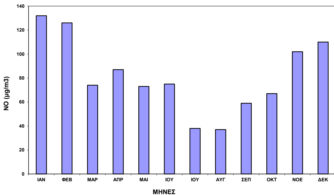
Σχήμα 2.13. Μέσες μηνιαίες τιμές NO στο σταθμό Πατησίων για το έτος 2016.
