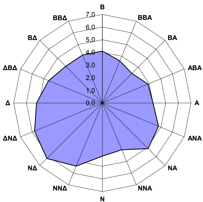
Σχήμα 3.6 Μέσες τιμές NO (σε \mu\text{g}/\text{m}^3 ) για το έτος 2016 στο σταθμό Πατησίων για κάθε διεύθυνση του ανέμου.
