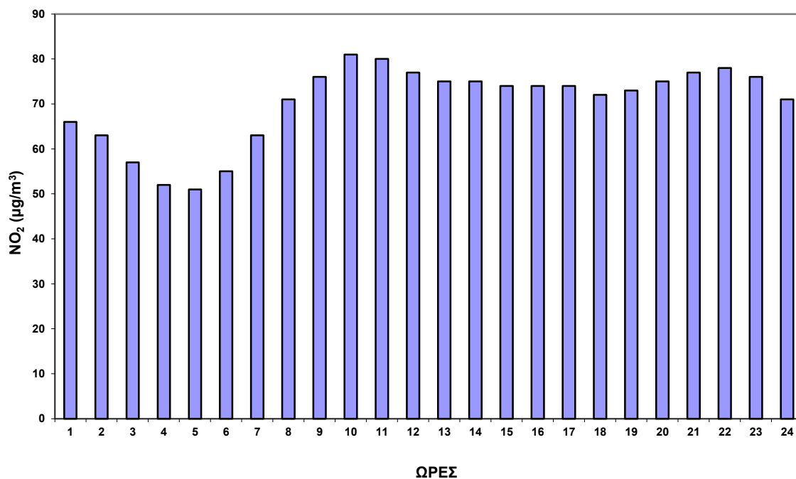
Σχήμα 2.22 Ωριαία μεταβολή NO₂ στο σταθμό Πατησίων για το έτος 2016.
