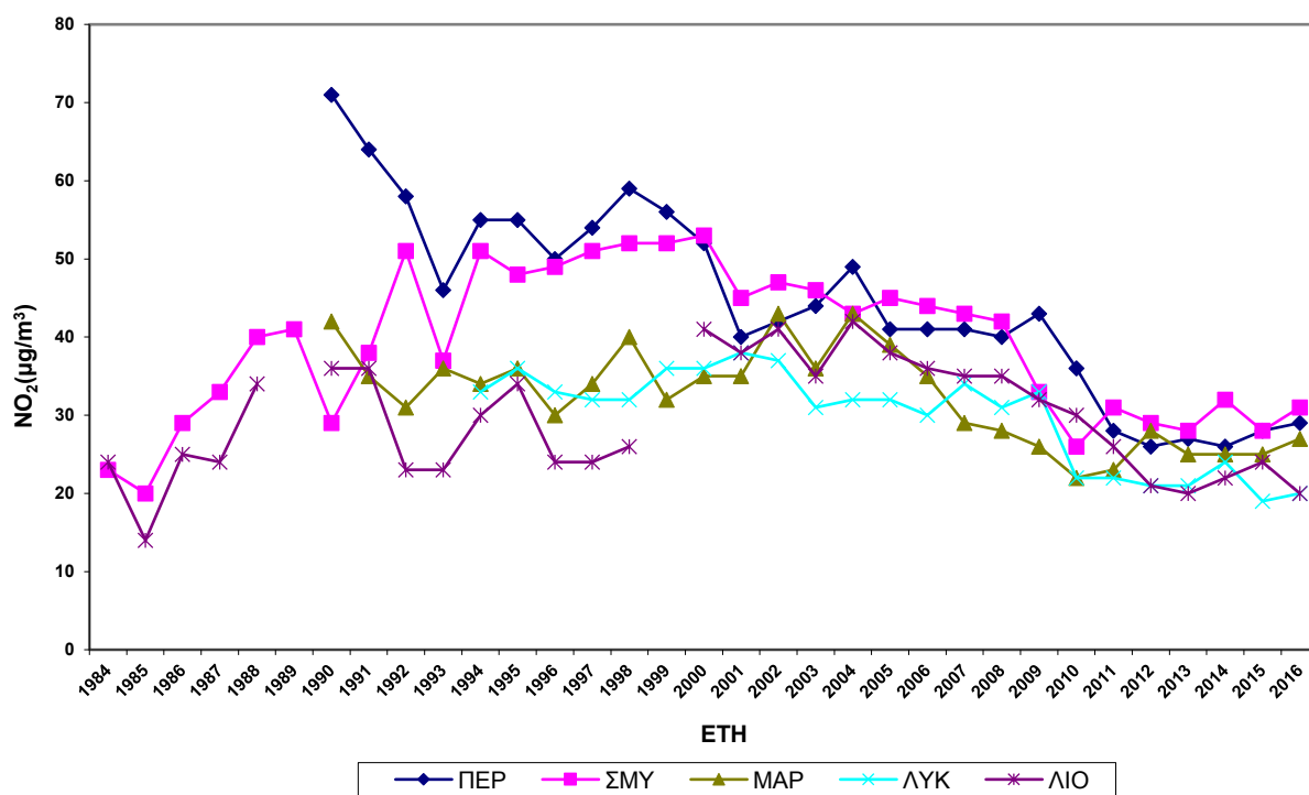
Σχήμα 2.5.β Διαχρονική μεταβολή μέσων ετήσιων τιμών \text{NO}_2 , σε \mu\text{g}/\text{m}^3 .
