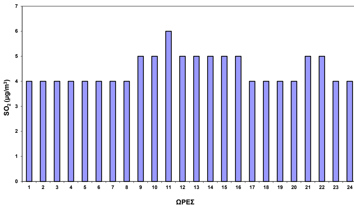
Σχήμα 2.19 Ωριαία μεταβολή SO 2 στο σταθμό Πατησίων για το έτος 2016.
