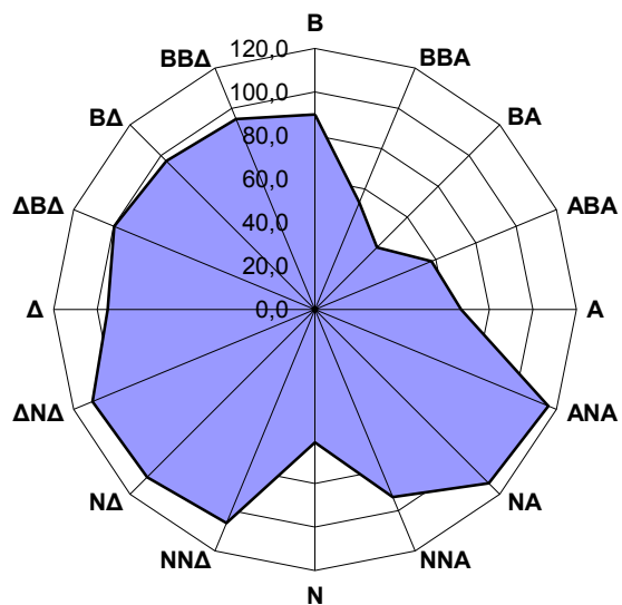
Σχήμα 3.6 Μέσες τιμές NO (σε \mu\text{g}/\text{m}^3 ) για το έτος 2016 στο σταθμό Πατησίων για κάθε διεύθυνση του ανέμου.
