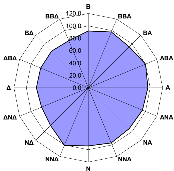
Σχήμα 3.4 Μέσες τιμές O 3 (σε μg/m 3 ) για το έτος 2016 στο σταθμό Θρακομακεδόνες για κάθε διεύθυνση του ανέμου.
