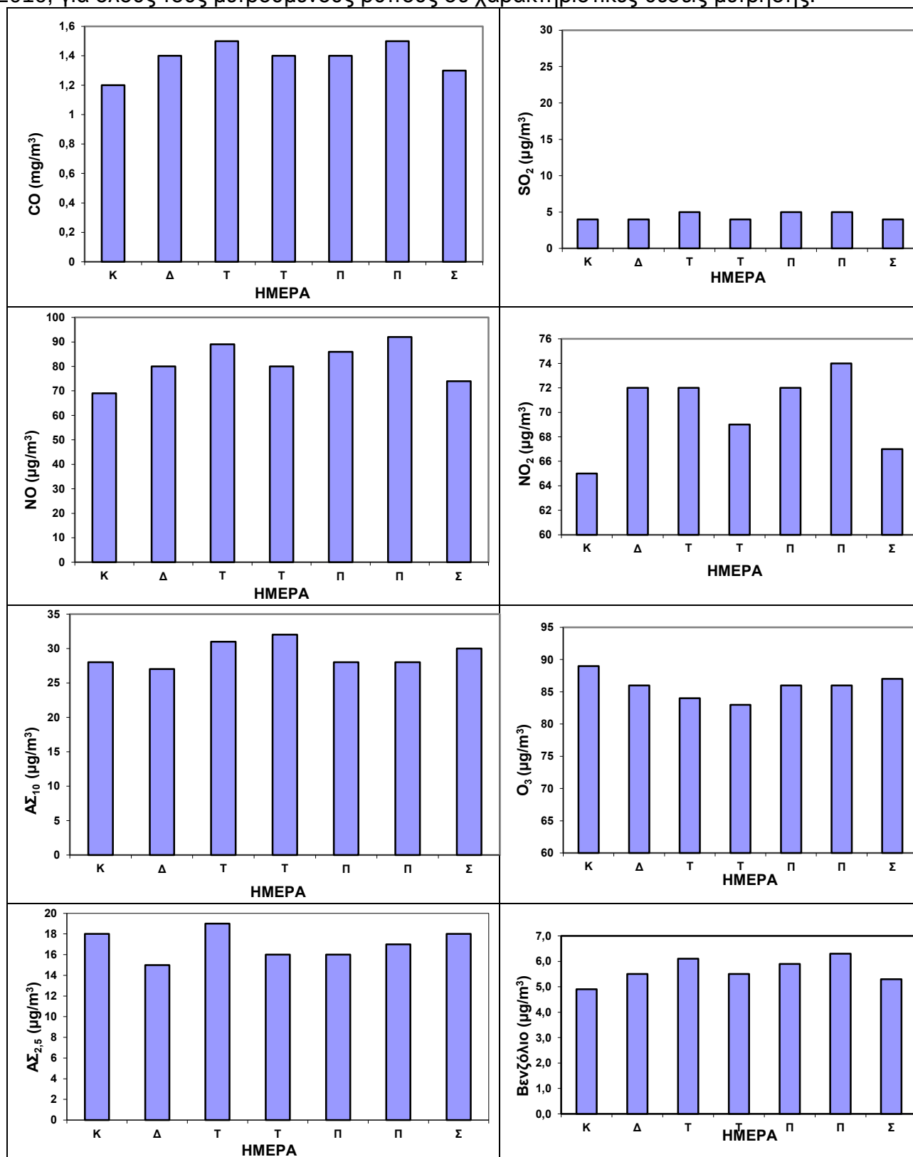
Σχήμα 2.17 Ημερήσια μεταβολή συγκεντρώσεων CO, NO, NO 2 , SO 2 και βενζολίου στο σταθμό Πατησίων, AΣ 10 , AΣ 2.5 στο σταθμό Λυκόβρυση και O 3 στο σταθμό Αγ. Παρασκευή για το έτος 2016.
