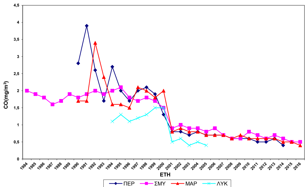
Σχήμα 2.1.β Διαχρονική μεταβολή μέσων ετησίων τιμών CO, σε mg/m 3 .
