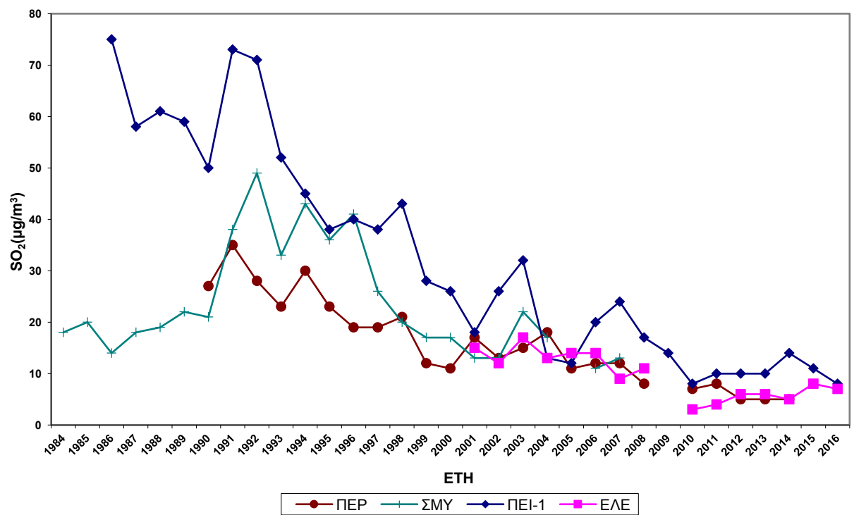
Σχήμα 2.2.β Διαχρονική μεταβολή μέσων ετήσιων τιμών SO_2 , σε \mu g/m^3 .
