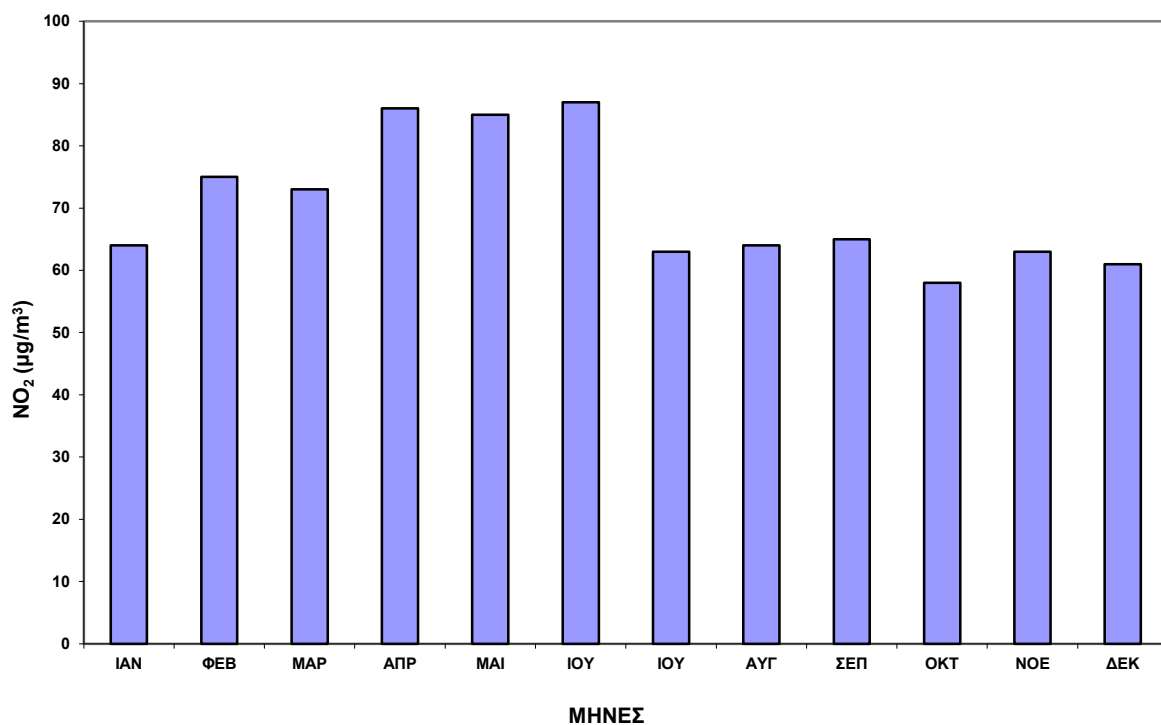
Σχήμα 2.12. Μέσες μηνιαίες τιμές NO 2 στο σταθμό Πατησίων για το έτος 2016.
