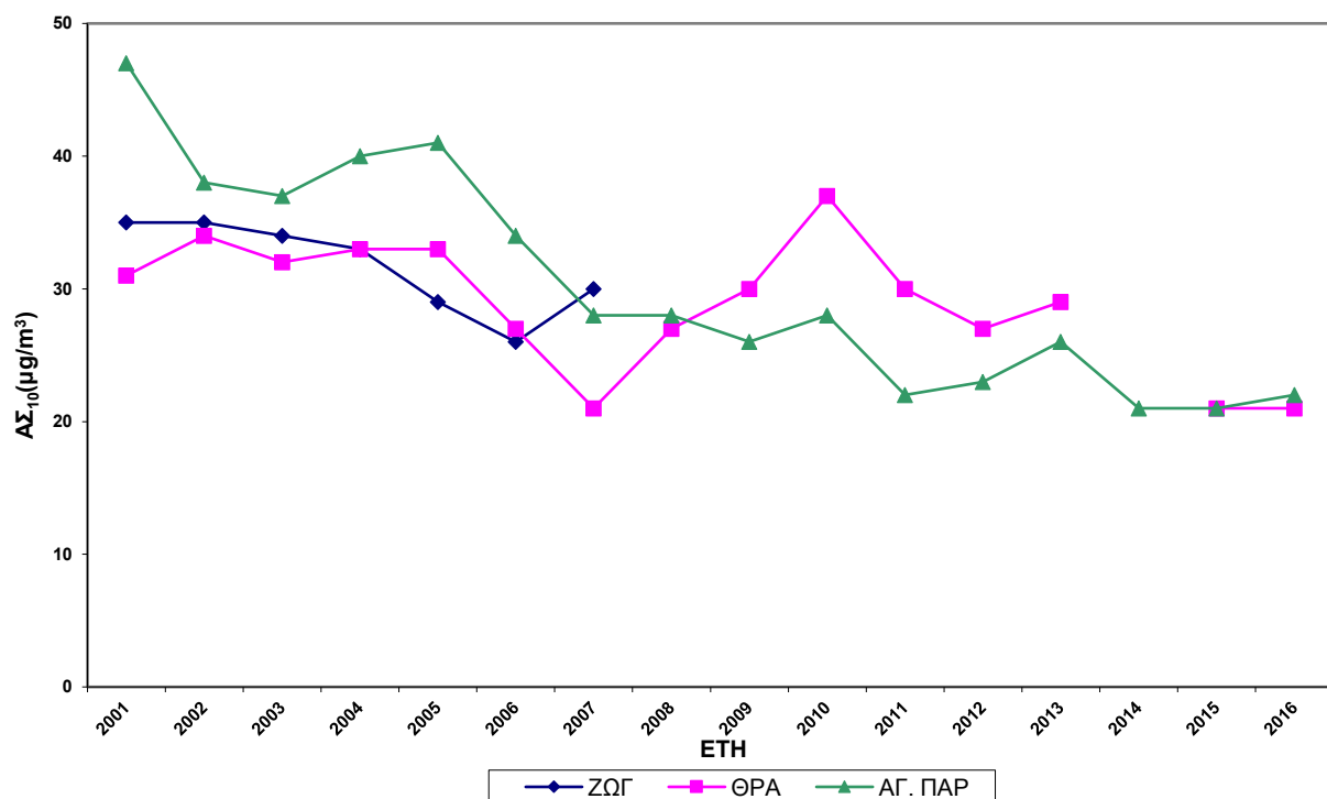
Σχήμα 2.7.β Διαχρονική μεταβολή μέσων ετήσιων τιμών AS_{10} , σε \mu g/m^3 .
