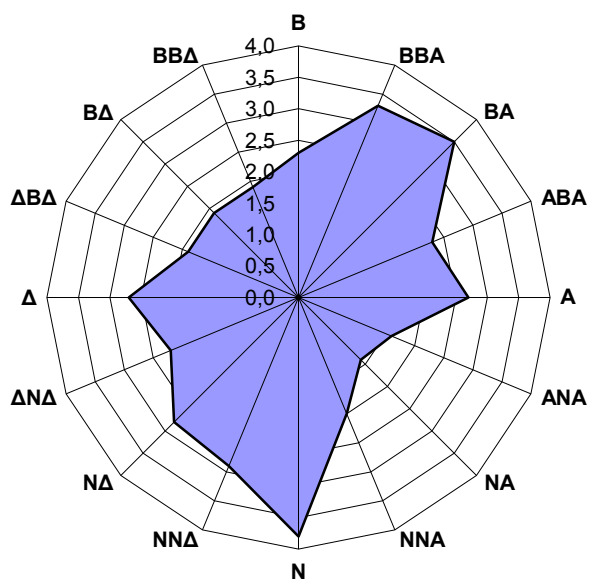
Σχήμα 3.2 Μέση ταχύτητα (σε m/s) ανά διεύθυνση ανέμου, στο σταθμό Πατησίων για το έτος 2016
