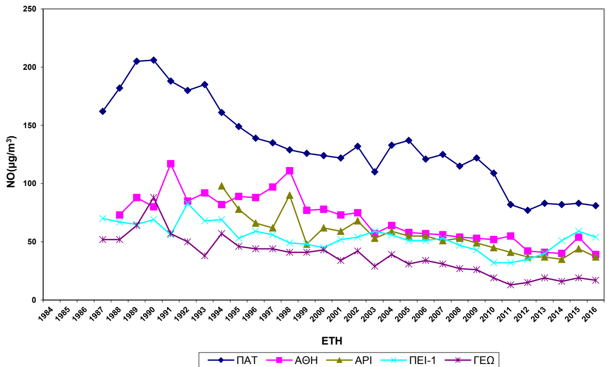
Σχήμα 2.4.α Διαχρονική μεταβολή μέσων ετήσιων τιμών NO, σε µg/m³.
