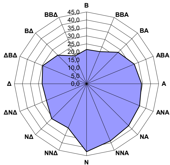
Σχήμα 3.8 Μέσες τιμές AS_{10} (σε \mu g/m^3 ) για το έτος 2016 στο σταθμό Λυκόβρυση για κάθε διεύθυνση του ανέμου.
