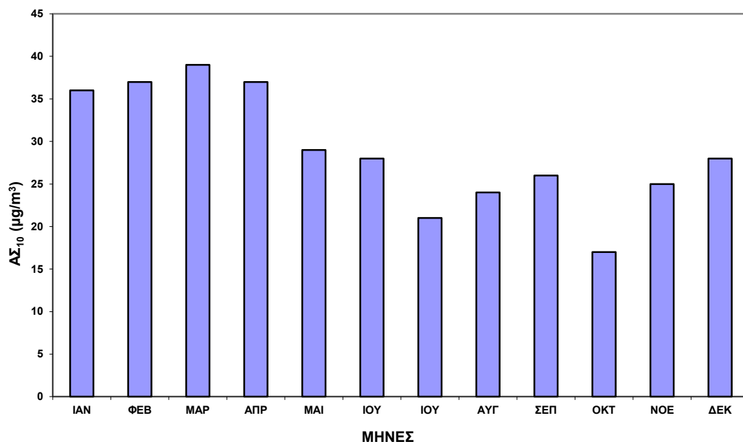
Σχήμα 2.14. Μέσες μηνιαίες τιμές ΑΣ 10 στο σταθμό Λυκόβρυση για το έτος 2016.
