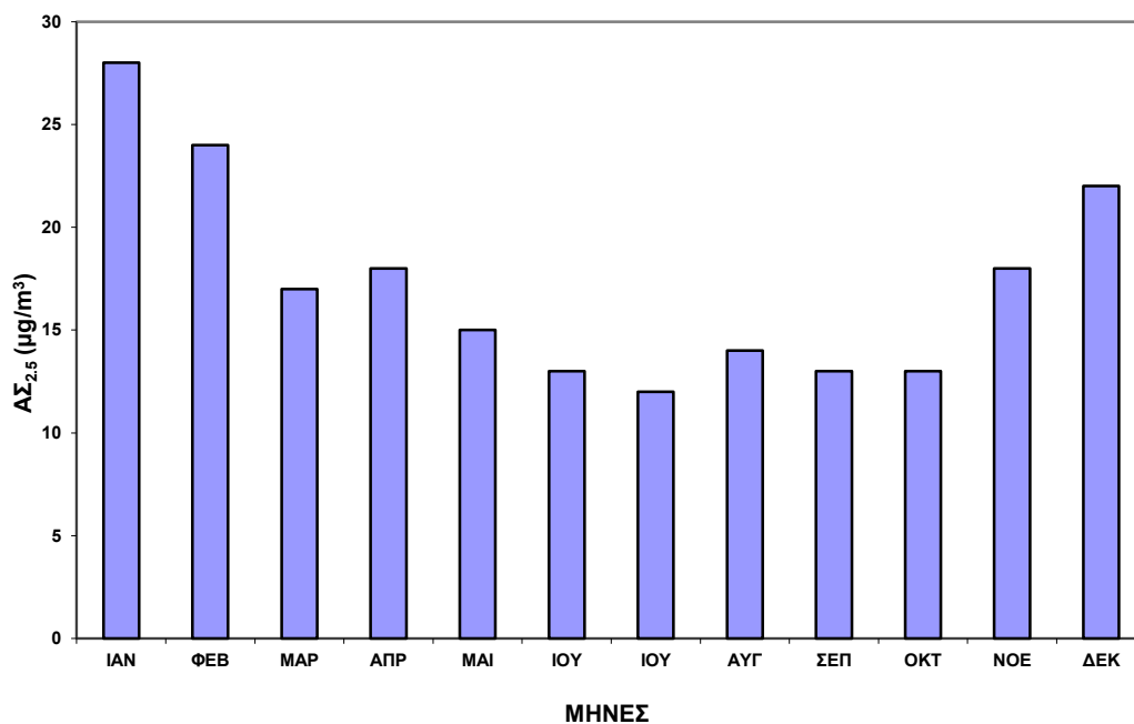
Σχήμα 2.15. Μέσες μηνιαίες τιμές ΑΣ 2,5 στο σταθμό Λυκόβρυση για το έτος 2016.
