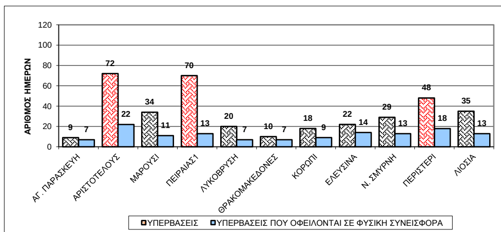
Σχήμα 5.1 Αριθμός ημερών για το 2016 με μέση ημερήσια τιμή ΑΣ 10 μεγαλύτερη από 50\mu\text{g}/\text{m}^3 (Με κόκκινο χρώμα σχεδιάζονται οι περιπτώσεις στις οποίες σημειώθηκε υπέρβαση του ορίου).
