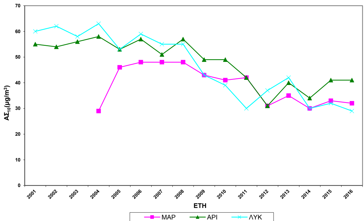
Σχήμα 2.7.α Διαχρονική μεταβολή μέσω των ετήσιων τιμών A\Sigma_{10} , σε \mu g/m^3 .
