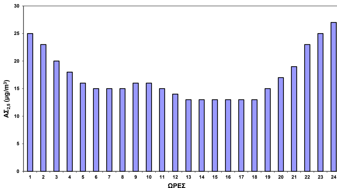
Σχήμα 2.25 Ωριαία μεταβολή AΣ 2,5 στο σταθμό Λυκόβρυση για το έτος 2016.
