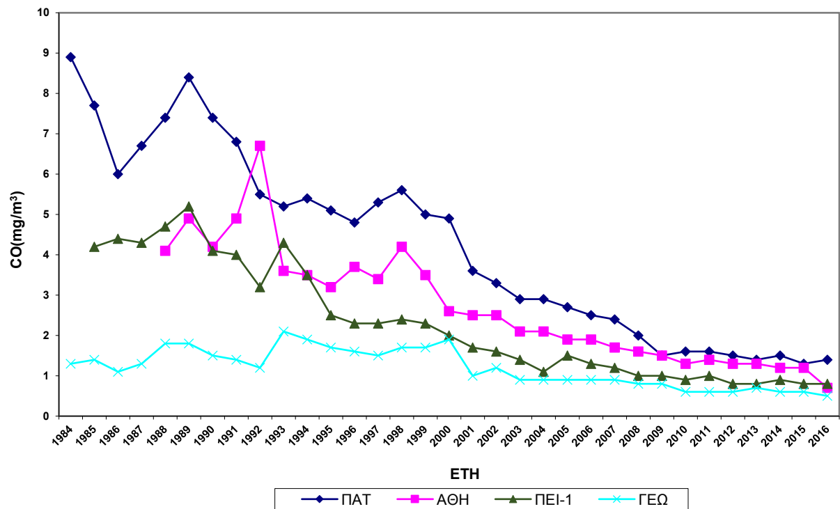
Σχήμα 2.1.α Διαχρονική μεταβολή μέσων ετησίων τιμών CO, σε mg/m 3 .
