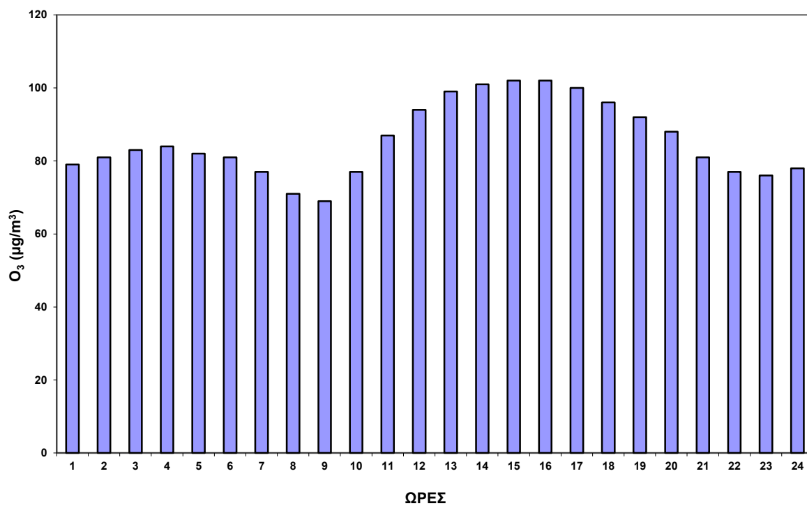
Σχήμα 2.23 Ωριαία μεταβολή O 3 στο σταθμό Αγ. Παρασκευή για το έτος 2016.
