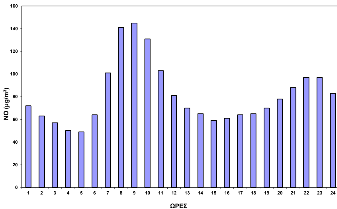
Σχήμα 2.20 Ωριαία μεταβολή NO στο σταθμό Πατησίων για το έτος 2016.
