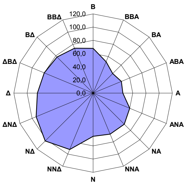
Σχήμα 3.3 Μέσες τιμές NO 2 (σε μg/m³) για το έτος 2016 στο σταθμό Πατησίων για κάθε διεύθυνση του ανέμου.
