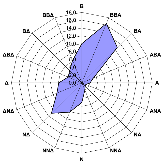
Σχήμα 3.1 Συχνότητες, επί τοις εκατό (%), των διευθύνσεων του ανέμου στο σταθμό Πατησίων για το έτος 2016.
