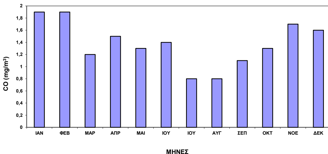
Σχήμα 2.9. Μέσες μηνιαίες τιμές \text{CO} στο σταθμό Πατησίων για το έτος 2016.
