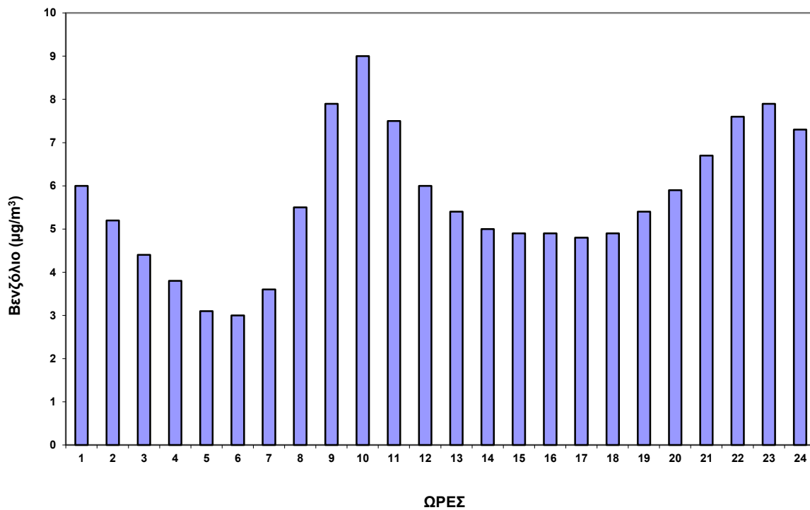
Σχήμα 2.21 Ωριαία μεταβολή βενζολίου στο σταθμό Πατησίων για το έτος 2016.
