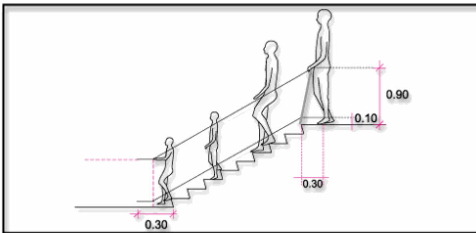
Εικόνα 26: Σχεδιασμός Βαθμίδων - Συνιστώμενοι τύποι χειρολαβών
